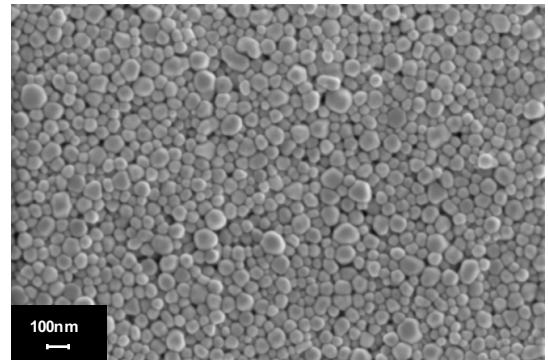
Nano Ag, HRSEM Image, x100,000
